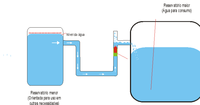
Figura 3 - Canalização da água da cisterna com sistema de boia.
